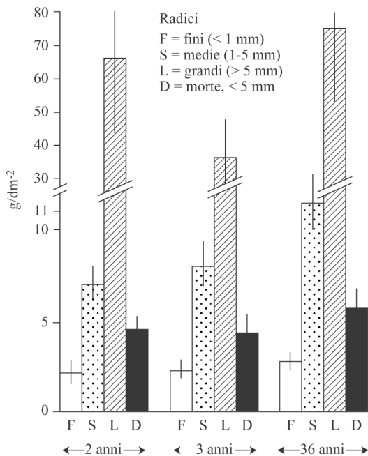
Fig. 8.26 - Biomassa radicale in popolamenti di Quercus coccifera , ripartita per classi di diametro delle radici in aree con diverse età di incendio (da TRABAUD, 1987).
