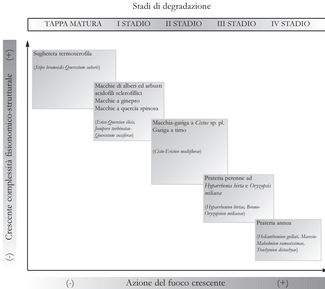
Fig. 8.55 - Schema della dinamica della vegetazione del piano termomediterraneo degli Erei meridionali (dati da: FURNARI, 1965; DE MARCO e FURNARI, 1976; BRULLO et al. , 1997a). La denominazione delle tipologie coinvolte nei diversi stadi della successione segue LA MANTIA et al. (2000, 2001); tra parentesi vengono riportate le corrispondenti unità fitosociologiche.
