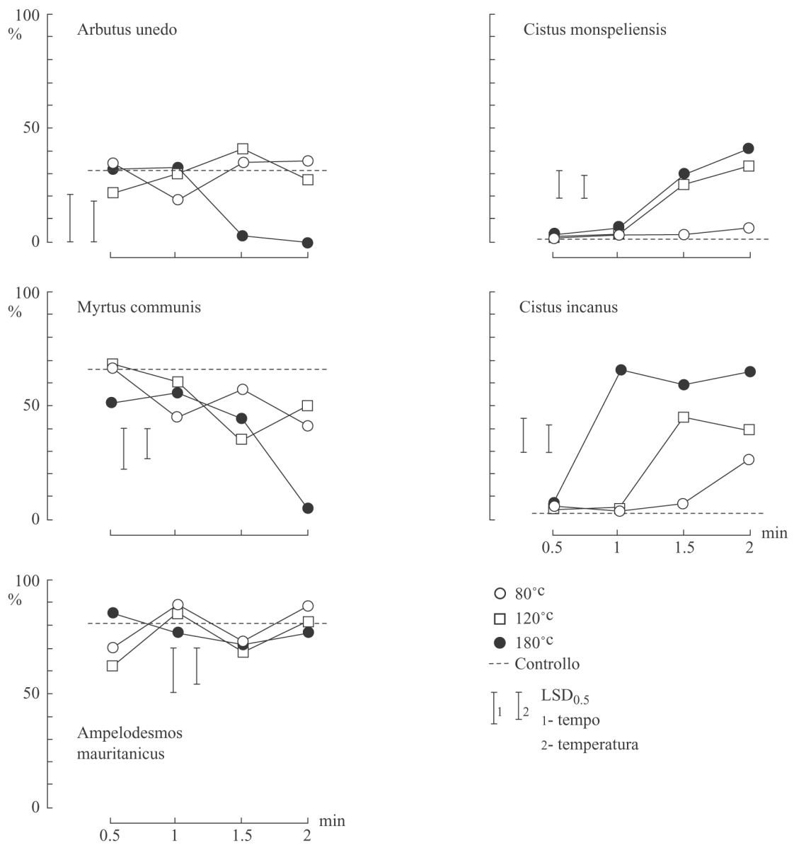
Fig. 2.13 - Percentuale di germinazione di alcune specie mediterranee in relazione alla temperatura e tempi di esposizione al calore (da MAZZOLENI, 1989).
