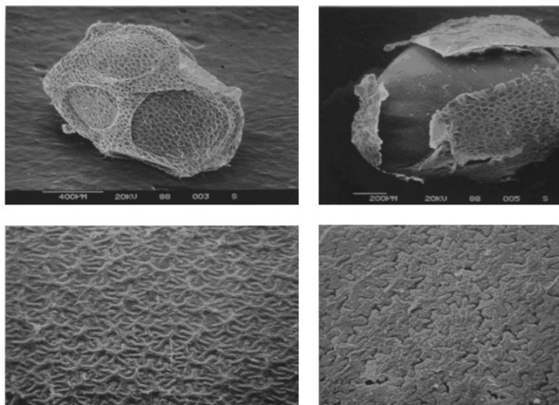
Fig. 2.14 - Effetto dell'esposizione al calore in semi di Cistus incanus . In alto a sinistra e a destra rispettivamente il seme prima e dopo il trattamento termico; in basso il corrispondente aspetto del tegumento interno (da ARONNE e MAZZOLENI, 1989).
