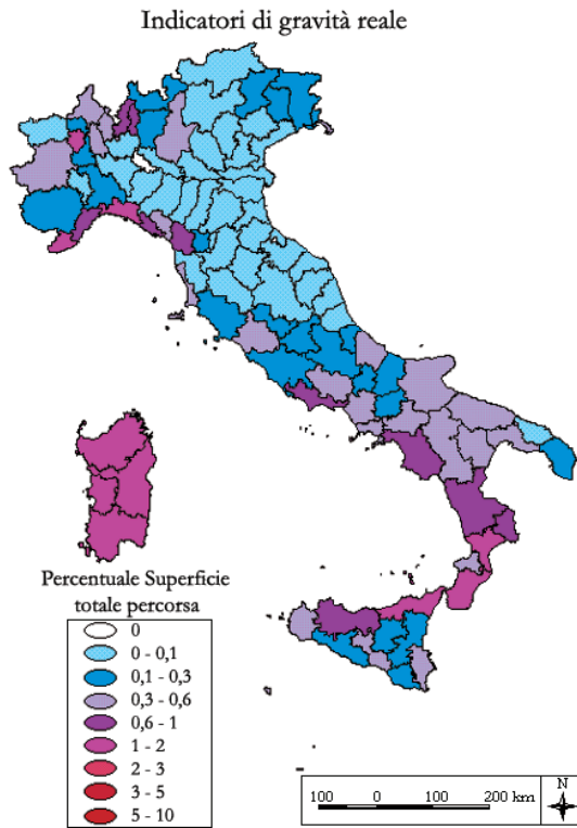
Fig. 4.32 - Carta del rapporto percentuale tra superficie totale percorsa annua (boscata e non boscata) e superficie territoriale provinciale.
