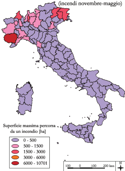
Fig. 4.30 - Carta della superficie massima percorsa da un incendio nel periodo invernale.
