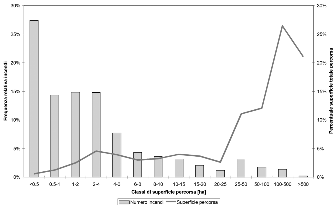
Fig. 4.7 - Percentuale di frequenze di incendio e superfici percorse, per classi di superficie in Italia (dal 1990 al 2000).
