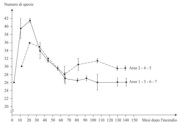
Fig. 8.20 - Variazione della Ricchezza floristica in aree a Quercus coccifera e Q. ilex del Sud della Francia (da TRABAUD, 1987).
