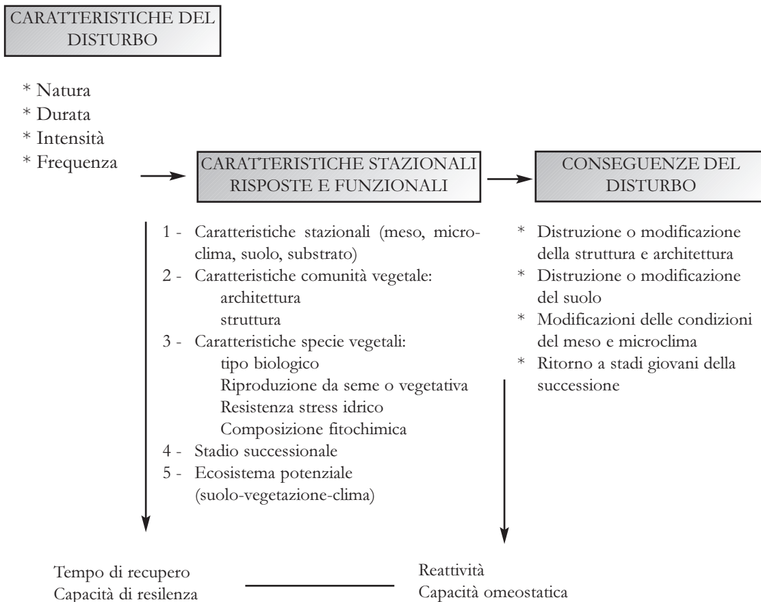
Fig. 8.1 - Fattori e conseguenze dell'incendio come disturbo (da BARBERO et al. , 1987).
