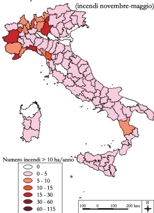
Fig. 4.26 - Carta del numero medio di incendi maggiori di 10 ha nel periodo invernale.
