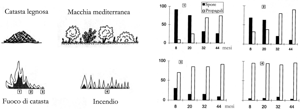
Fig. 8.16 - Frequenza post-incendio delle diverse strategie di riproduzione nelle principali specie di briofite di un'area a vegetazione mediterranea dell'Italia meridionale sottoposte a diverse intensità di incendio (da ESPOSITO et al. , 1999).
