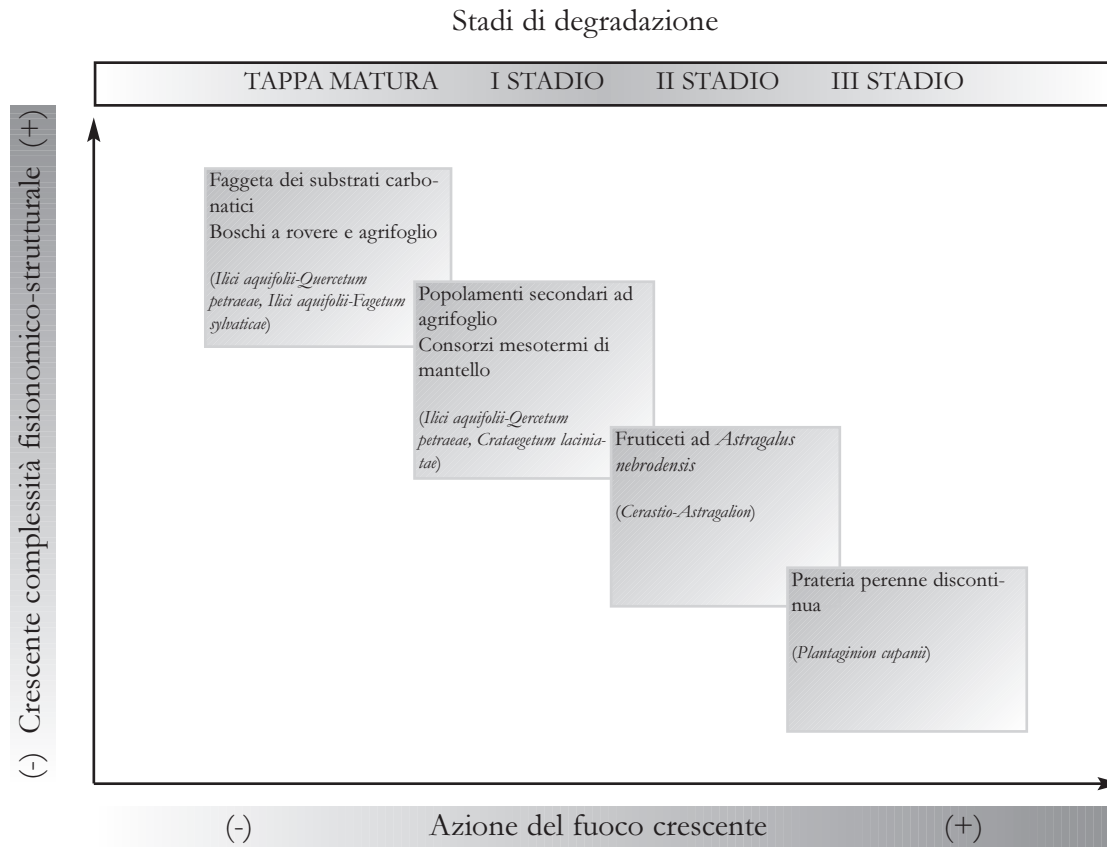
Fig. 8.59 - Schema della dinamica della vegetazione del piano supramediterraneo delle Madonie (dati da: HOFFMANN, 1960; RAIMONDO, 1983; BRULLO, 1984a; RAIMONDO et al. , 1994). La denominazione delle tipologie coinvolte nei diversi stadi della successione segue LA MANTIA et al. (2000, 2001); tra parentesi vengono riportate le corrispondenti unità fitosociologiche.
