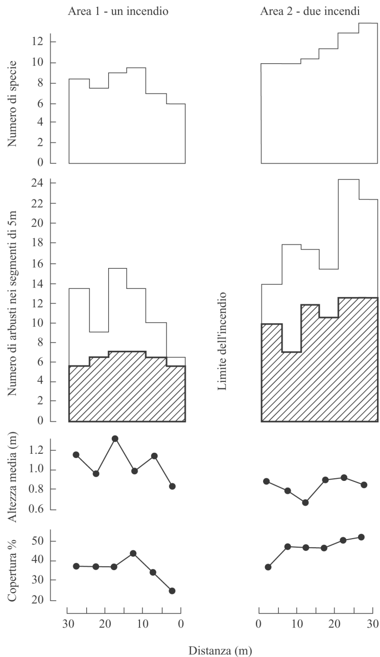
Fig. 8.7 - Differenze nella struttura e ricchezza floristica di due aree boscate del Myall Lakes National Park (Australia) sottoposte a diverse frequenze di incendio (da FOX e FOX, 1986).
