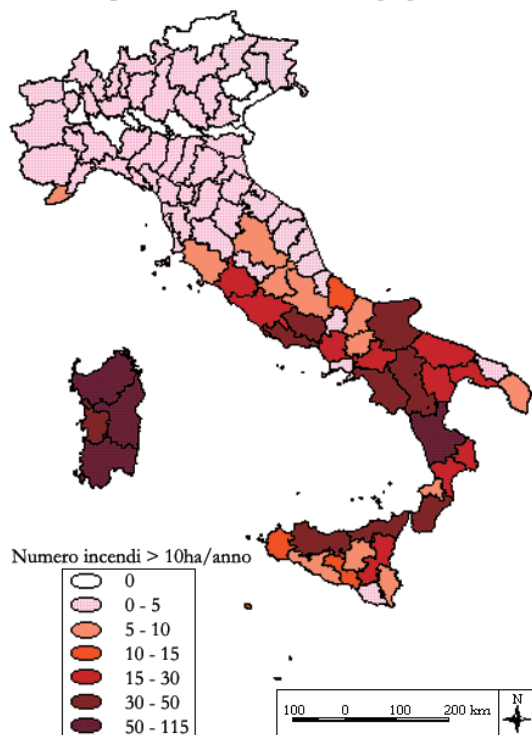
Fig. 4.18 - Carta del numero medio di incendi maggiori di 10 ha nel periodo estivo.
