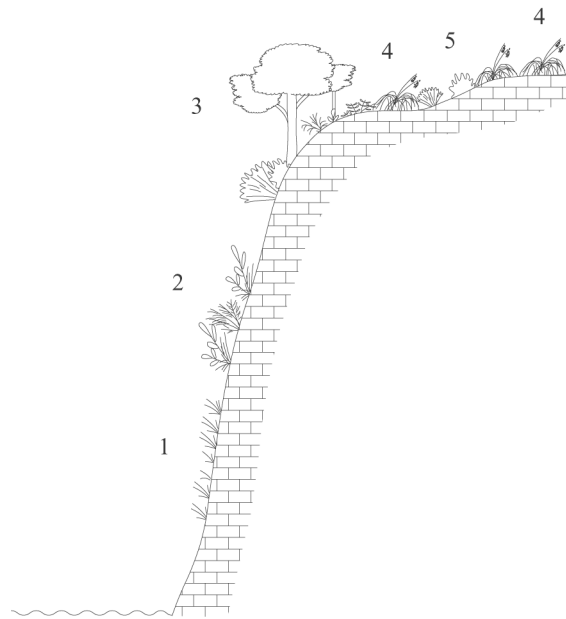
Fig. 8.46 - Transetto della vegetazione del promontorio di Portovenere ad Est rispetto al centro abitato: 1. Aggr. a Crithmum maritimum , 2. Rhamno alaterni-Euphorbietum dendroidis , 3. Junipero oxycedri-Pinetum halepensis , 4. Coronillo valentinae-Ampelodesmetum mauritanicae myrtetosum communis , 5. Ruto chalepensis-Thymetum vulgare (da VAGGE, 2000).
