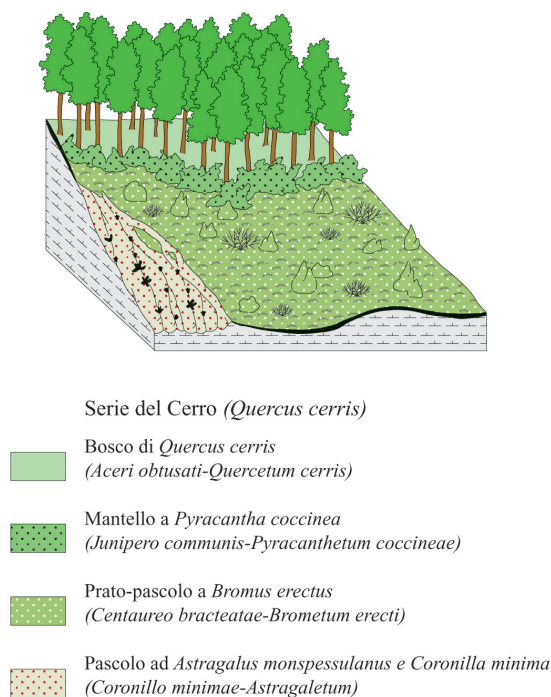
Fig. 8.27 - La serie di vegetazione del cerro, sui terreni marnoso-arenacei, dell'Umbria e delle Marche (da BIONDI et al. , 1990).
