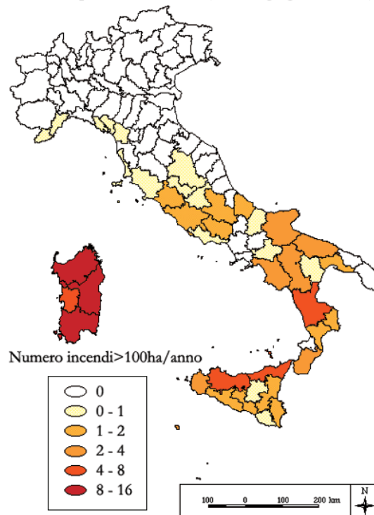
Fig. 4.17 - Carta del numero medio di incendi maggiori di 100 ha nel periodo estivo.
