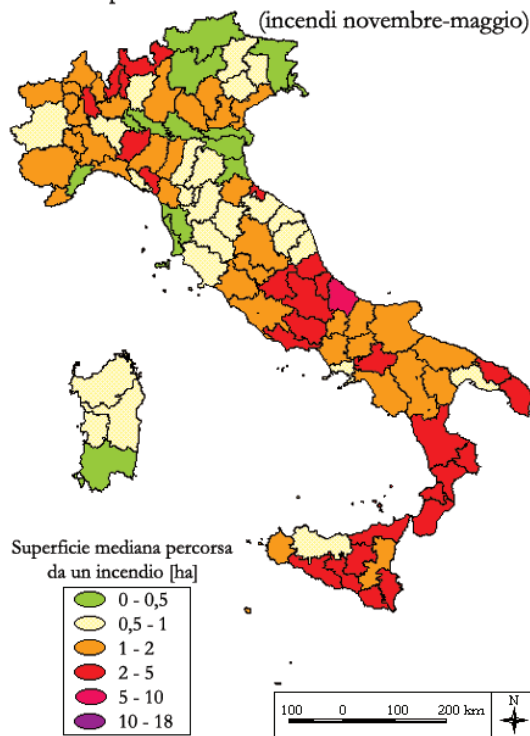
Fig. 4.28 - Carta della superficie mediana percorsa da un incendio nel periodo invernale.
