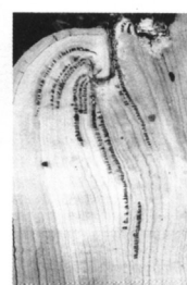
Fig. 2.2 - Datazioni di cicatrici di incendio in un esemplare di Pinus ponderosa delle foreste dell'Arizona (da SCHWEINGRUBER, 1996).
