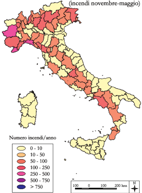
Fig. 4.24 - Carta del numero medio di incendi nel periodo invernale.
