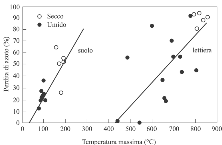
Fig. 2.3 - Volatilizzazione dell'azoto dai compartimenti del suolo e della lettiera in relazione alla temperatura massima raggiunta durante un incendio (da DEBANO et al. , 1977).
