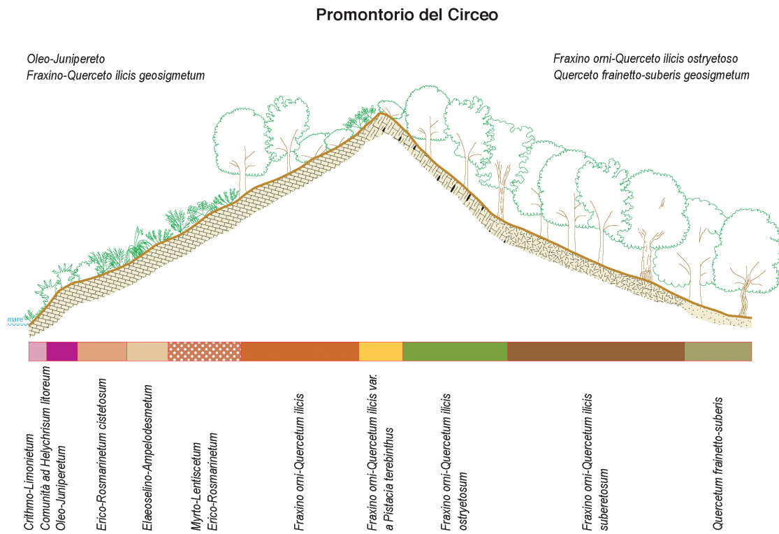
Fig. 8.32 - Paesaggio vegetale del Promontorio del Circeo.
