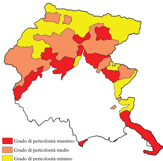
Fig. 8.40 - Carta della pericolosità degli incendi boschivi (da Regione Autonoma Friuli-Venezia Giulia, 1998).
