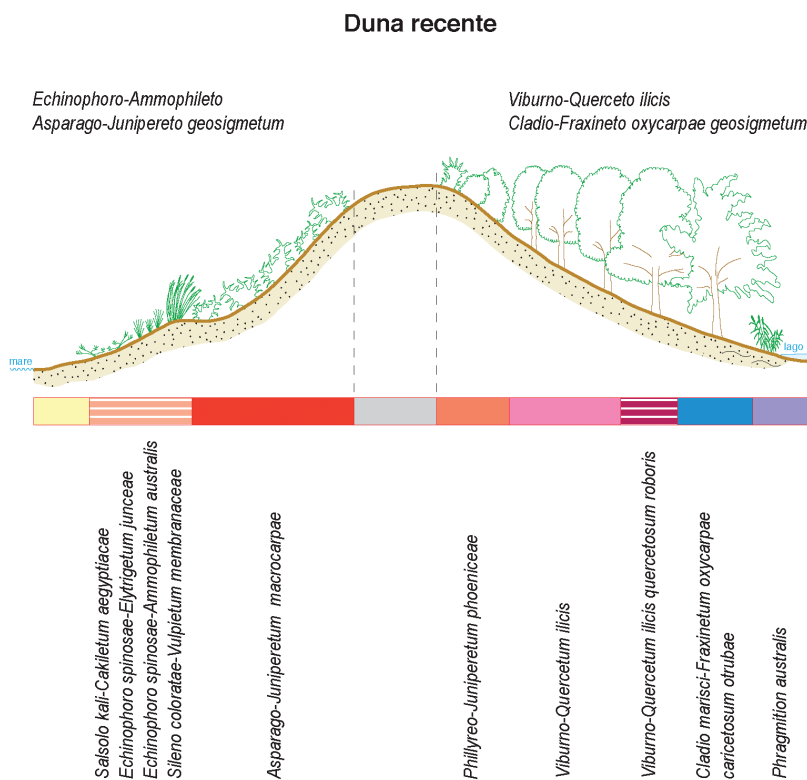
Fig. 8.33 - Paesaggio vegetale della duna recente (Parco Nazionale del Circeo).
