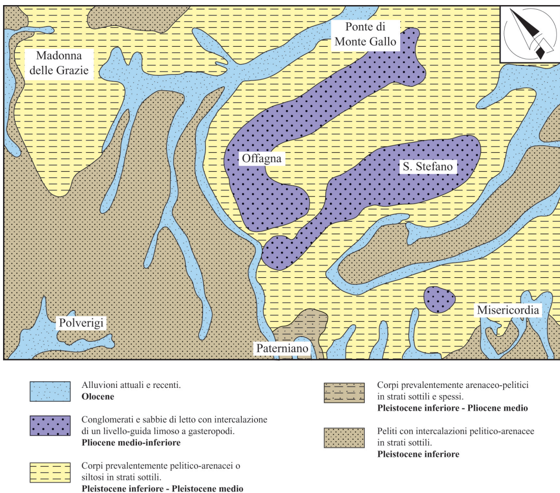
Fig. 8.29 - Schema geologico del settore collinare anconetano.
