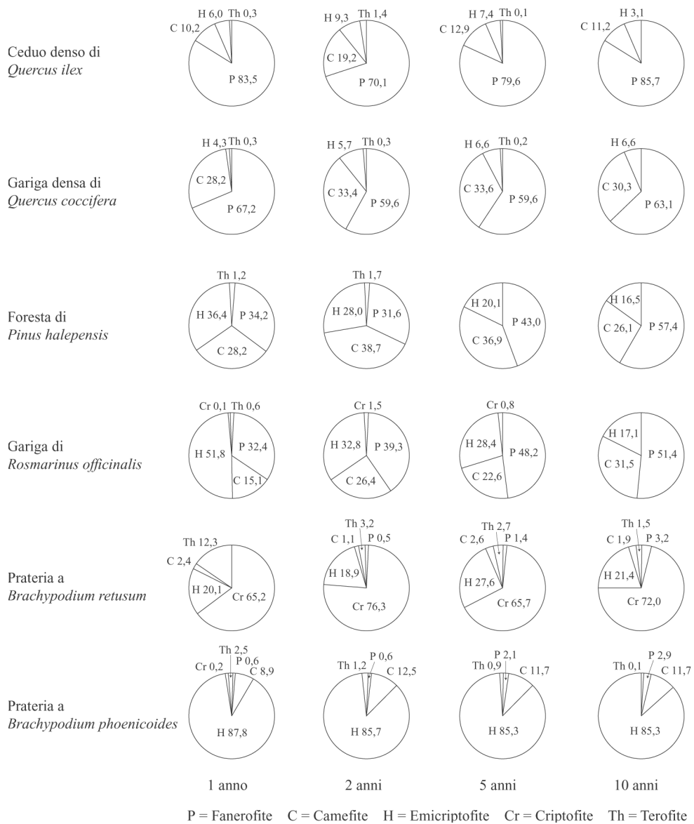
Fig. 8.23 - Cambiamenti post-incendio delle forme biologiche di differenti comunità vegetali del Sud della Francia (da TRABAUD, 1987).
