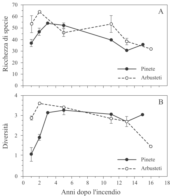
Fig. 8.13 - Ricchezza specifica (A) e indice di diversità di Shannon (B) in vari stadi successionali post-incendio di cisteti e pinete della Spagna (da FARACO et al. , 1993).
