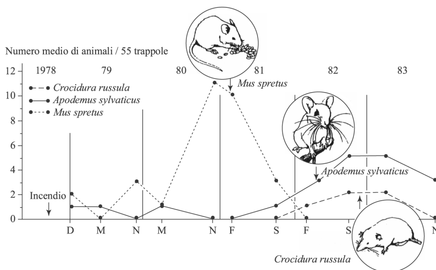
Fig. 2.19 - Successione post-incendio di micro-roditori in una macchia bassa incendiata. Sulle ordinate è riportato il numero di individui per trappole) (da PRODON et al. , 1987).
