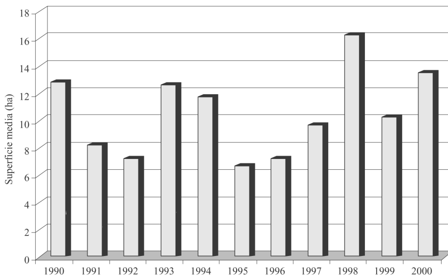
Fig. 4.1 - Superfici medie percorse da un incendio in Italia.
