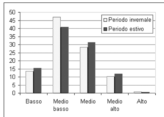
Fig. 4.39 - Ripartizione percentuale del territorio italiano in funzione del rischio di incendio.
