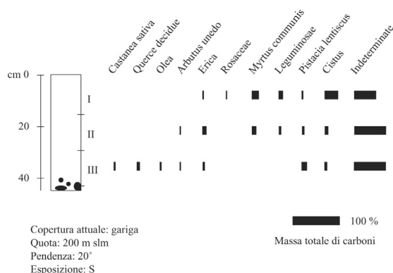
Fig. 2.1 - Analisi quali-quantitativa dei carboni in un suolo di Punta Tresino (Parco Nazionale del Cilento e Vallo di Diano) (da DI PASQUALE e MAZZOLENI, 2001).
