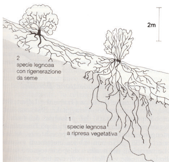
Fig. 2.12 - Morfologia e profondità dell'apparato radicale in specie a ripresa vegetativa (1) e da seme (2) (da DE LILLIS, 1995).
