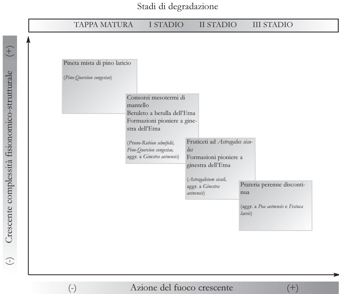
Fig. 8.60 - Schema della dinamica della vegetazione del piano supramediterraneo dell'Etna (dati da: HOFFMANN, 1960; BRULLO et al. , 1996a, 1999). La denominazione delle tipologie coinvolte nei diversi stadi della successione segue LA MANTIA et al. (2000, 2001); tra parentesi vengono riportate le corrispondenti unità fitosociologiche.
