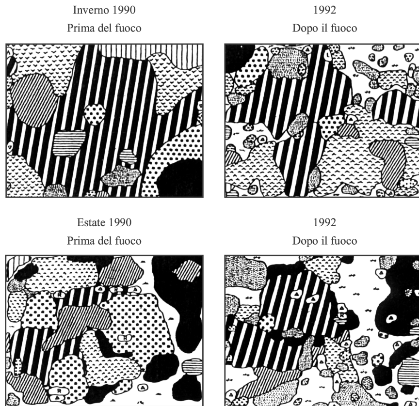
Fig. 8.4 - Mappe di copertura della vegetazione in aree soggette a fuochi estivi ed invernali (da MAZZOLENI e ESPOSITO, 1993)
