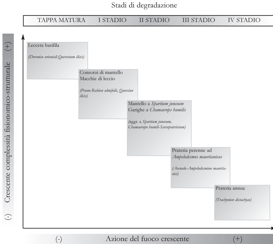
Fig. 8.57 - Schema della dinamica della vegetazione basifila del piano mesomediterraneo degli Iblei (dati da: BARBAGALLO et al. , 1979; BARTOLO et al. , 1990). La denominazione delle tipologie coinvolte nei diversi stadi della successione segue LA MANTIA et al. (2000, 2001); tra parentesi vengono riportate le corrispondenti unità fitosociologiche.
