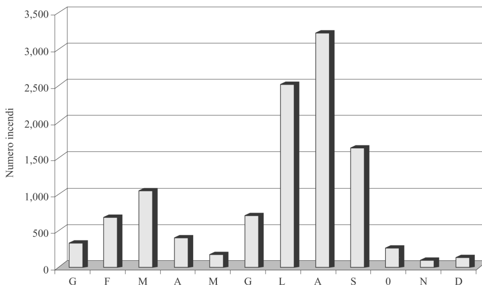
Fig. 4.2 - Frequenze medie mensili di incendio in Italia (dal 1990 al 2000).
