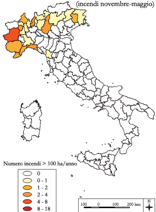
Fig. 4.25 - Carta del numero medio di incendi maggiori di 100 ha nel periodo invernale.
