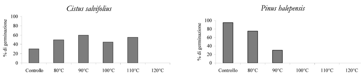
Fig. 2.15 - Effetto della temperatura sulla germinazione di plantule di due specie mediterranee adattate al fuoco ( Cistus salvifolius e Pinus halepensis ) (modificato da HANLEY e FENNER, 1998).
