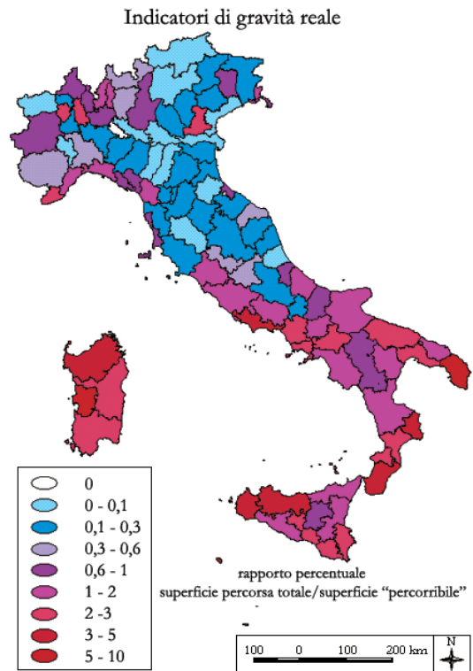
Fig. 4.34 - Carta del rapporto percentuale tra superficie totale percorsa annua (boscata e non boscata) e superficie provinciale "percorribile" (boscata e non boscata).
