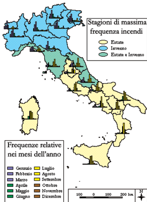
Fig. 4.11 - Frequenze mensili di incendio nelle Regioni italiane (anni 1990-2000). Gli istogrammi riportano le frequenze relative nei mesi rispetto alla frequenza annua di ogni Regione.
