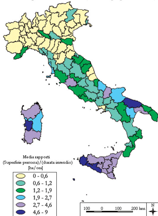
Fig. 4.21 - Carta della media dei rapporti tra superficie percorsa e durata degli incendi nel periodo estivo.
