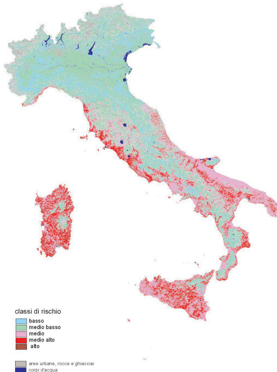
Fig. 4.37 - Carta del rischio di incendi boschivi in Italia nel periodo estivo.
