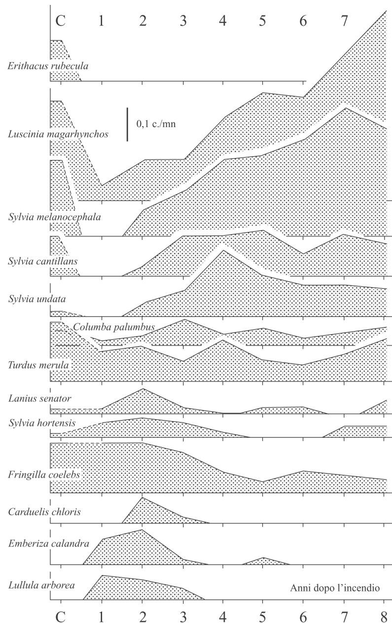
Fig. 2.20 - Successione post-incendio dell'avifauna in una macchia bassa incendiata. Sulle ordinate è riportato il numero di individui per trappole (da PRODON et al. , 1987).
