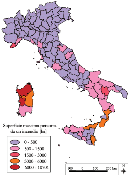
Fig. 4.22 - Carta della superficie massima percorsa da un incendio nel periodo estivo.
