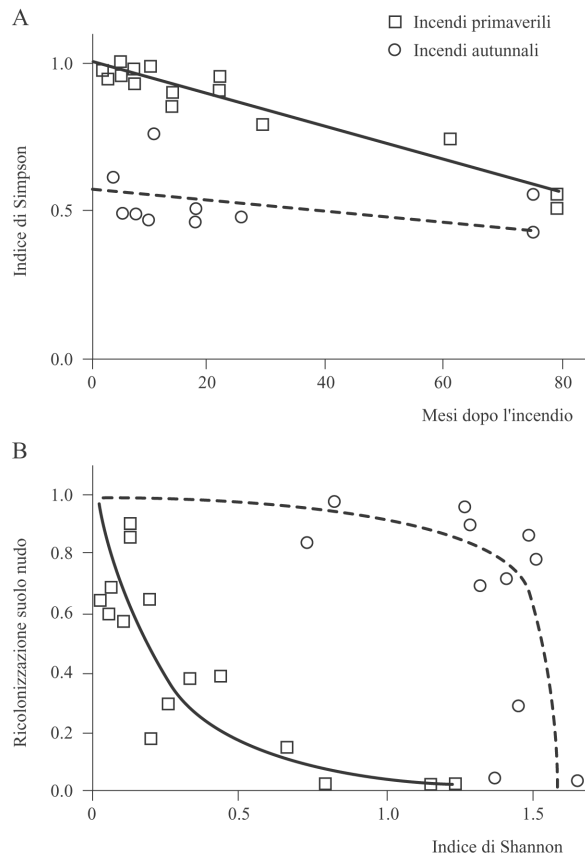
Fig. 8.5 - Variazione post-incendio dell'indice di Simpson (A) e di Shannon (B) calcolati sui valori di copertura delle specie legnose in una comunità ad Ulex europaeus (da CASAL, 1987).
