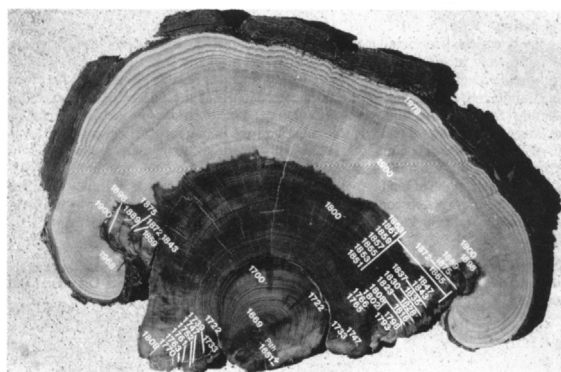
Fig. 2.1 - Analisi quali-quantitativa dei carboni in un suolo di Punta Tresino (Parco Nazionale del Cilento e Vallo di Diano) (da DI PASQUALE e MAZZOLENI, 2001).
