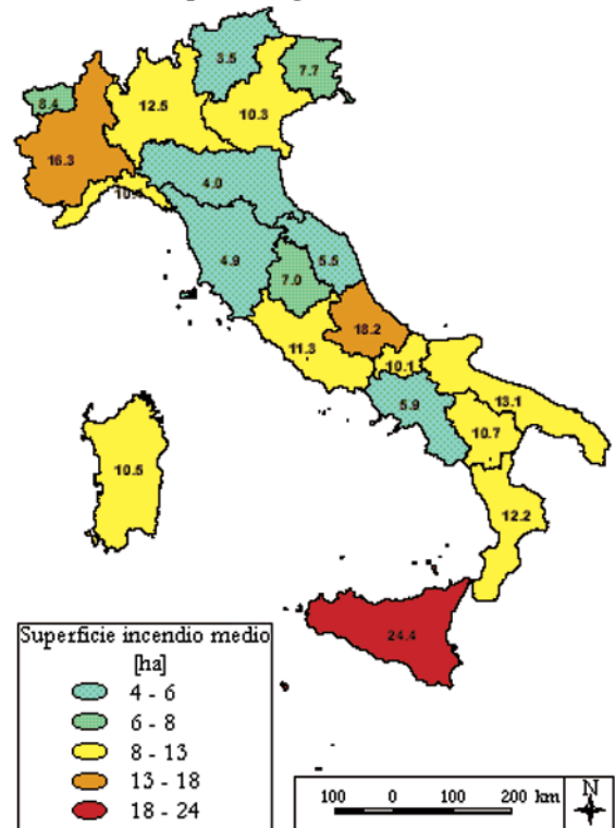
Fig. 4.13 - Superficie dell'incendio medio nelle Regioni italiane (anni 1990-2000).
