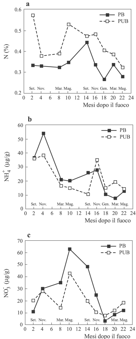
Fig. 2.4 - Variazioni delle concentrazioni di azoto totale (a), ammonio (b) e nitrato alla superficie del suolo (0-3 cm) dopo incendio nelle foreste di pino d'Aleppo (PB = suolo incendiato; PUB = suolo non incendiato) (da KUTIEL e NAVEH, 1987).
