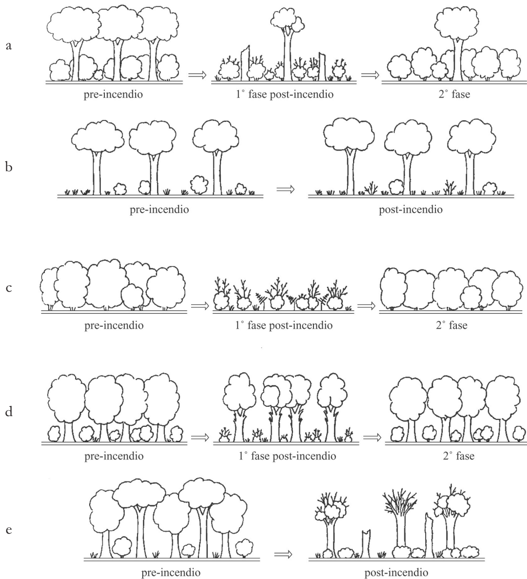
Fig. 8.50 - Variazioni di struttura dopo l'incendio: a - pineta con abbondante sottobosco, b - pineta con sottobosco scarso, c - macchia, d - bosco di sclerofille sempreverdi, e - bosco misto di sclerofille sempreverdi e pini (da BARBERIS et al. , 1994).
