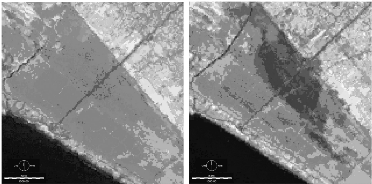
Figura 7.2. Immagini telerilevate dal satellite LANDSAT della pineta di Castel Fusano (Roma), prima (luglio 1998) e subito dopo (fine luglio 2000) l'incendio di cui alla Figura 7.1. L'immagine è stata ottenuta dalla fusione falsocolore delle bande TM5, TM4 e TM3 (fonte: CHIRICI et al. , 2003).
