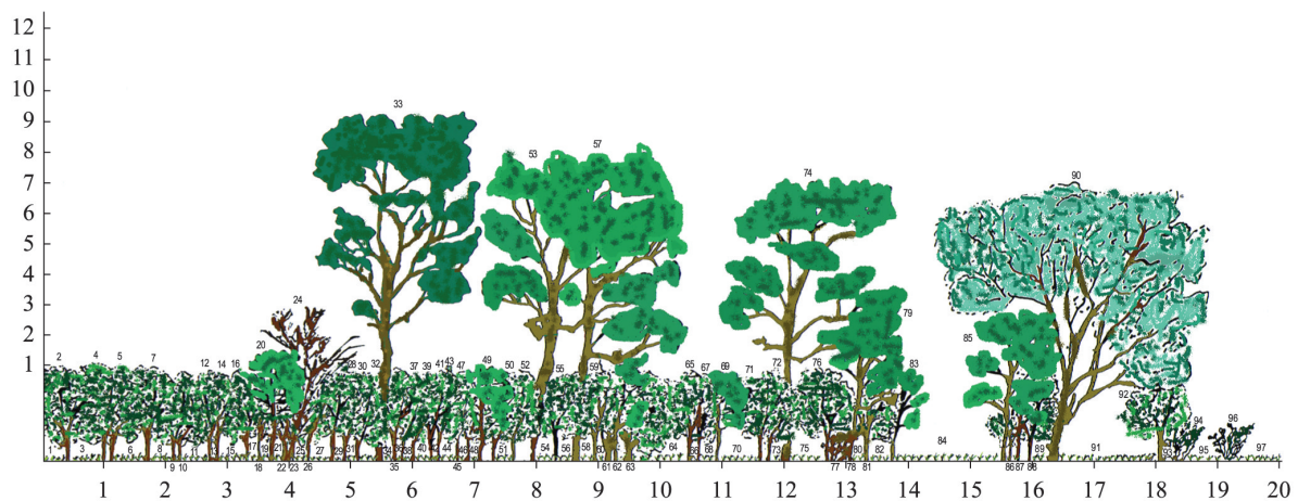
Fig. 8.37 - Transetto realizzato all'interno di un'area permanente di studio del rimboschimento del Monte Conero (da BAIOTTO et al. , 1996)
