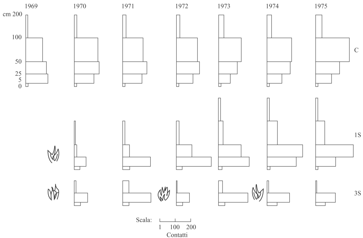
Fig. 8.6 - Variazioni nello sviluppo dei diversi strati della vegetazione in aree sottoposte a diverse frequenze di incendio (da GODRON et al. , 1981).
