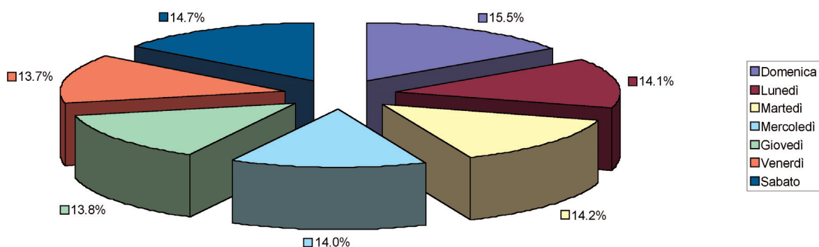
Fig. 4.5 - Frequenze relative di incendio nei giorni della settimana in Italia (dal 1990 al 2000).
