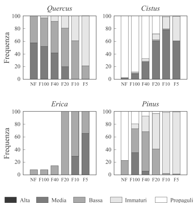
Fig. 8.17 - Risultati di una simulazione secondo il modello FATE di specie rappresentative di quattro diversi tipi funzionali. NF=No fire; F100=incendio ogni 100 anni; F40=incendio ogni 40 anni; F20= incendio ogni 20 anni; F10=incendio ogni 10 anni; F5=incendio ogni 5 anni. Sull'asse delle Y è riportata la frequenza di ricorrenza in 500 anni di simulazione (da PAUSAS, 1999).
