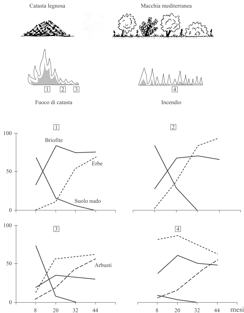
Fig. 8.8 - Cambiamenti nella copertura del suolo nudo, briofite, erbe e arbusti in aree a macchia mediterranea sottoposte a differenti intensità di incendio (da ESPOSITO et al. , 1999).
