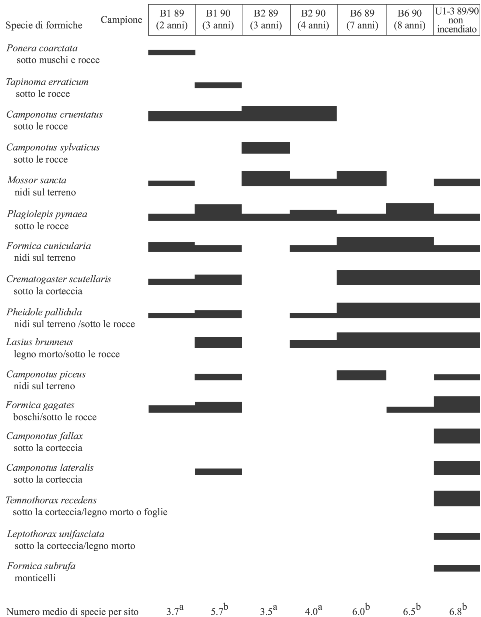
Fig. 2.21 - Frequenze in popolazioni di formiche ricorrenti in aree con diversa storia di incendio (da ALTENBURG et al. , 1993).
