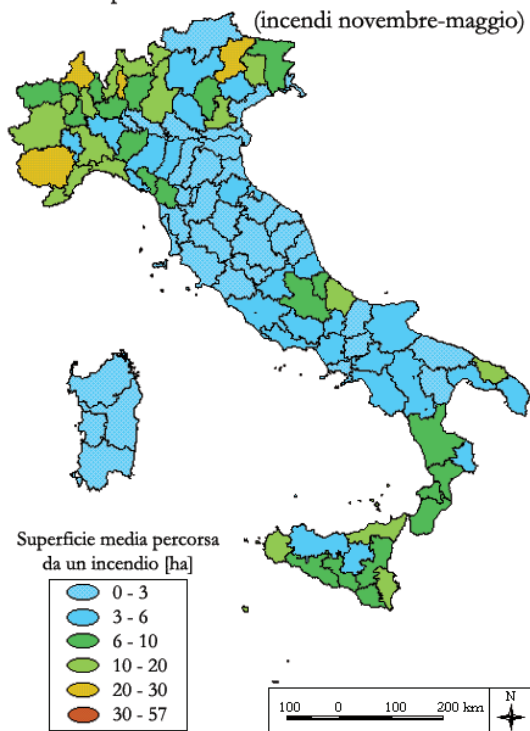
Fig. 4.27 - Carta della superficie media percorsa da un incendio nel periodo invernale.
