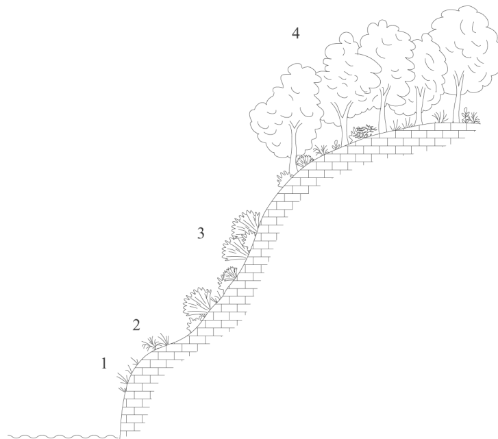
Fig. 8.45 - Transetto della vegetazione del promontorio di Montemarcello presso Punta Bianca: 1. aggr. a Crithmum maritimum , 2. aggr. a Crithmum maritimum variante a Dianthus sylvestris , 3. Rhamno alaterni-Euphorbietum dendroidis , 4. Viburno tini-Quercetum ilicis (da VAGGE, 2000).
