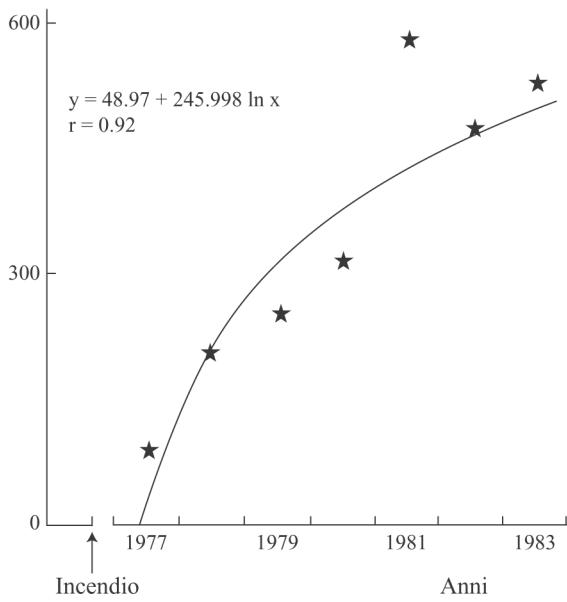
Fig. 8.25 - Cambiamenti post-incendio della biomassa epigea in una comunità a gariga (da ARIANOTSOU-FARAGGITAKI, 1984).
