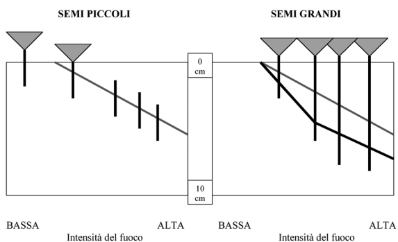
Fig. 2.16 - Relazione tra la grandezza del seme e la risposta all'intensità del fuoco (modificato da BOND, 1998).
