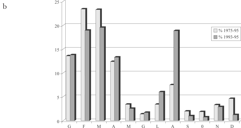
Fig. 8.41 - Correlazione tra diagrammi termoudometrici di alcune località del Friuli-Venezia Giulia (a) e distribuzione degli incendi, espressa in percentuale, secondo i mesi dell'anno (b); questi ultimi dati si riferiscono al periodo 1975-1995 e sono desunti da Regione Autonoma Friuli-Venezia Giulia (1998).
