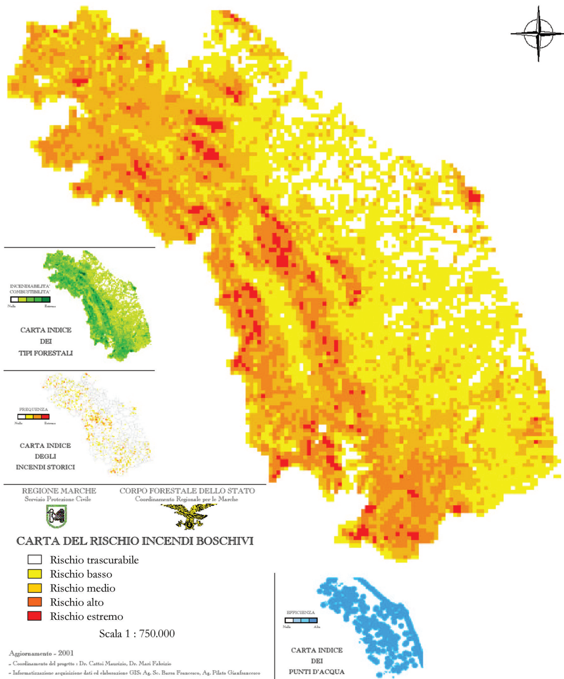
Fig. 8.35 - Carta del rischio di incendi boschivi nelle Marche (per gentile concessione del Coordinamento regionale Marche del Corpo Forestale dello Stato).
