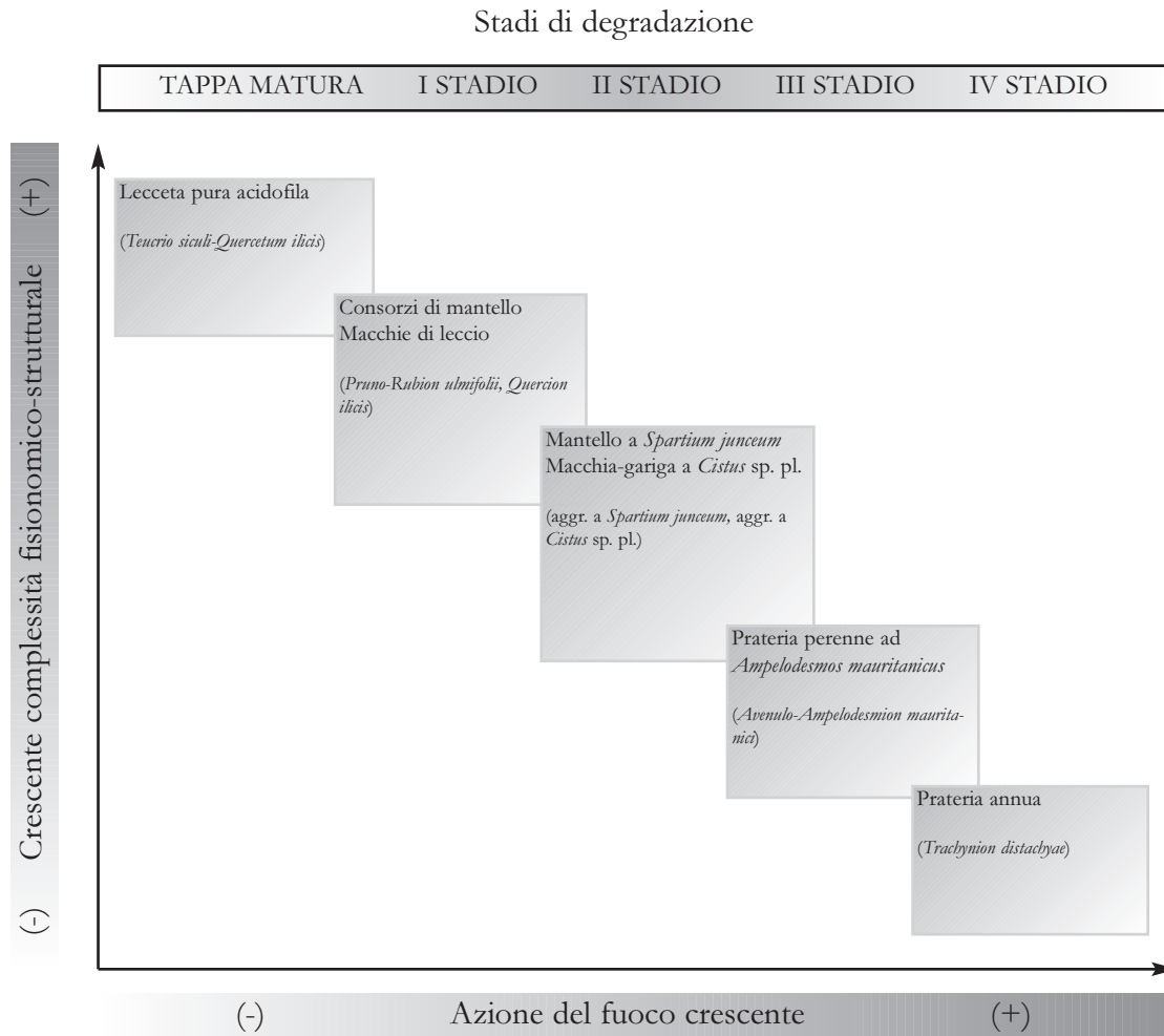
Fig. 8.58 - Schema della dinamica della vegetazione acidofila del piano mesomediterraneo degli Nebrodi (dati da: GENTILE, 1969; BRULLO e MARCENÒ, 1985; BARTOLO et al. , 1990). La denominazione delle tipologie coinvolte nei diversi stadi della successione segue LA MANTIA et al. (2000, 2001); tra parentesi vengono riportate le corrispondenti unità fitosociologiche.
