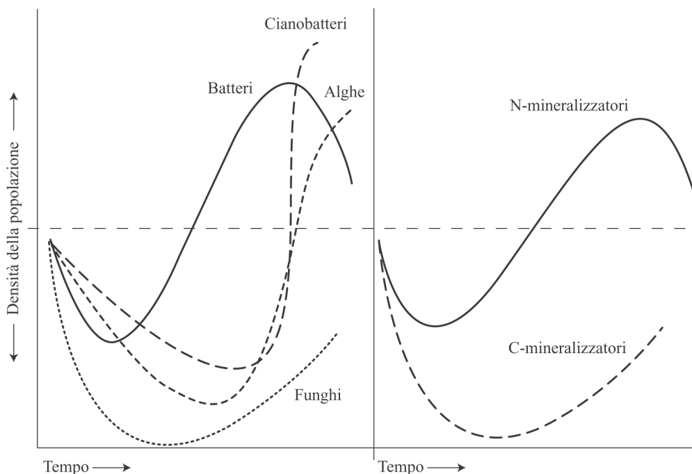
Fig. 2.6 - Modelli di comportamento della componente microbica dopo incendio del suolo (da CARBALLAS et al. , 1993).
