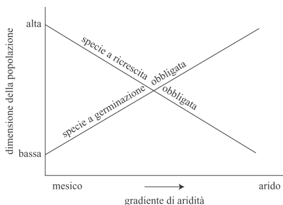
Fig. 2.11 - Andamenti delle popolazioni di specie a ricrescita obbligatoria e di specie a germinazione obbligatoria in relazione al gradiente di aridità del sito (da KEELY, 1986).
