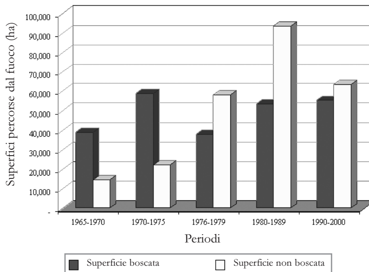
Fig. 3.2 - Superfici medie annue boscate e non boscate percorse dal fuoco in Italia dal 1965 al 2000.
