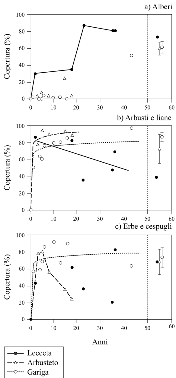
Fig. 8.14 - Dinamica post-incendio della copertura di specie arboree, arbustive, suffrutici ed erbe in tre differenti comunità vegetali (da FERRAN e VALLEJO, 1998).
