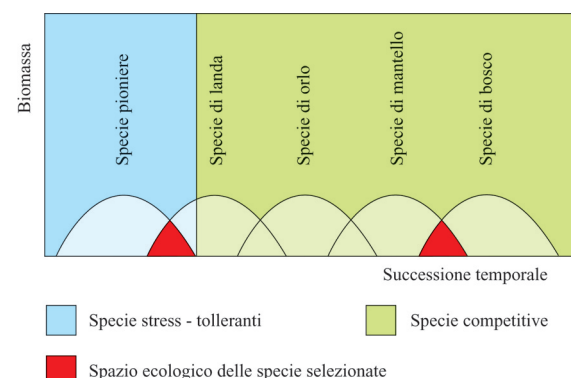
Fig. 8.42 - Successione temporale nelle serie di vegetazione e campi di esistenza delle specie stress-tolleranti e di quelle competitive (da POLDINI et al. , 2001).
