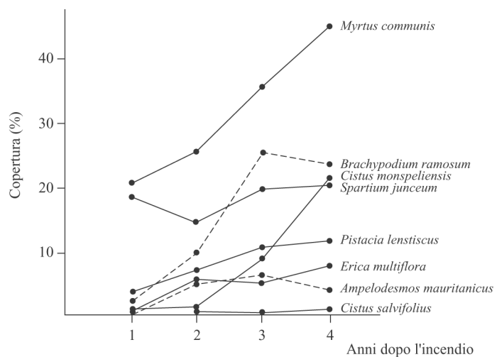
Fig. 8.22 - Variazioni post-incendio nella copertura delle principali specie della macchia mediterranea costiera dell'Italia meridionale (da DE LILLIS e TESTI, 1990).
