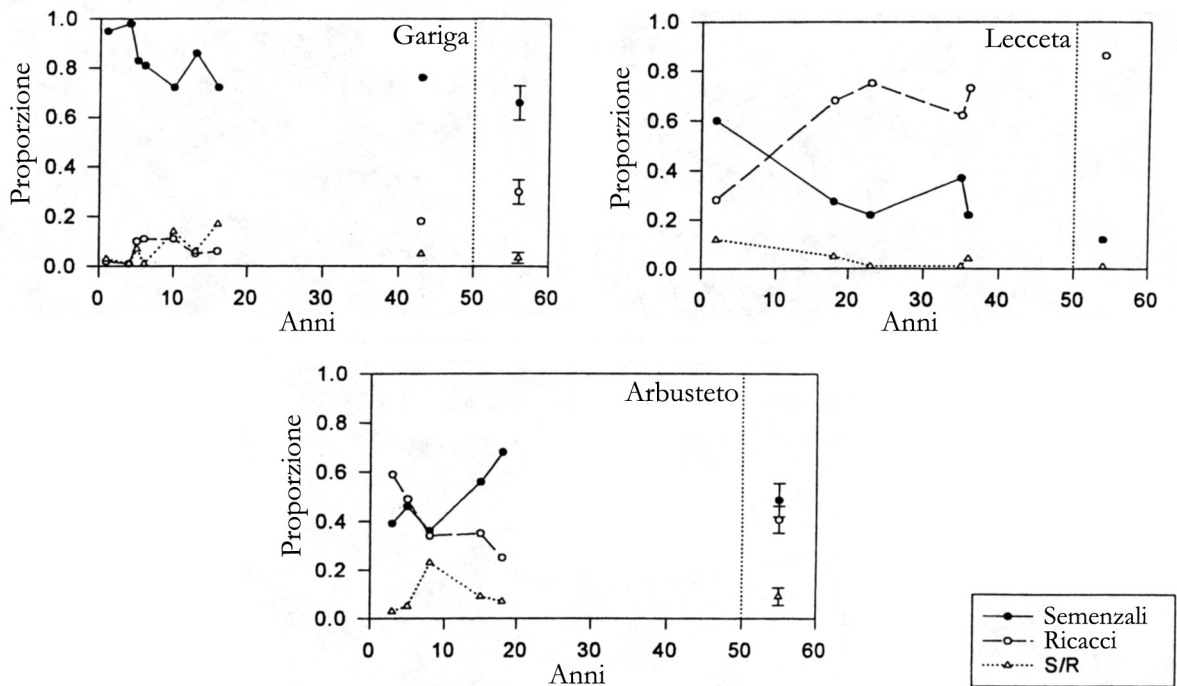
Fig. 8.15 - Dinamica post-incendio delle diverse strategie rigenerative (rigenerazione da seme, vegetativa o entrambe) in tre differenti comunità vegetali (da FERRAN et al. , 1998).
