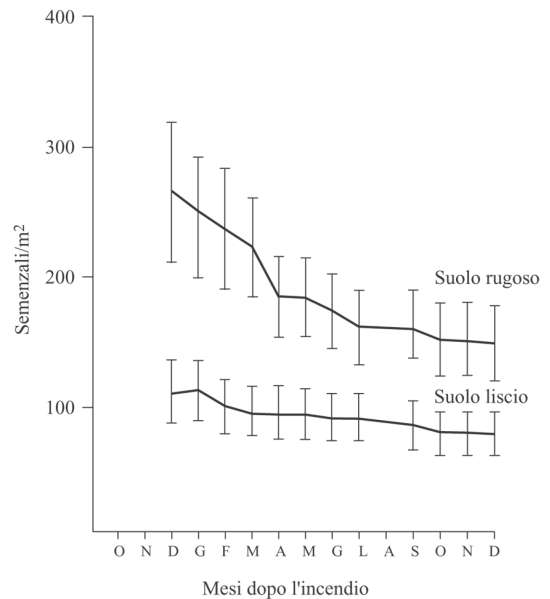
Fig. 8.10 - Cambiamenti post-incendio del numero di plantule di Ulex europaeus in relazione alla microtopografia (da PUENTES et al. , 1985).
