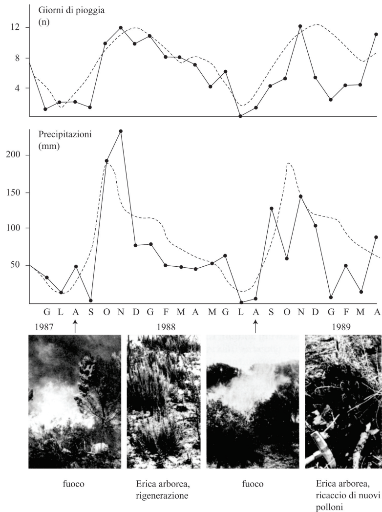
Fig. 8.2 - Il numero di giorni di pioggia e l'ammontare delle precipitazioni per il periodo 1987-1989 ed effetti sull'attecchimento post-incendio di germogli di Erica arborea da rigenerazione vegetativa.
