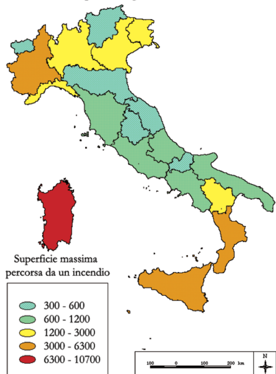
Fig. 4.14 - Superficie massima percorsa da un incendio nelle Regioni italiane (anni 1990-2000).
