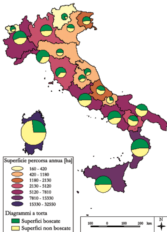
Fig. 4.10 - Superfici percorse dal fuoco medie annue nelle Regioni italiane (anni 1990-2000). La dimensione dei diagrammi a torta è proporzionale alla superficie totale percorsa.
