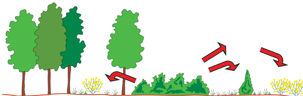
Fig. 8.28 - Il funzionamento del mantello di vegetazione nei processi di occupazione delle praterie non utilizzate (da BIONDI et al. , 1988).
