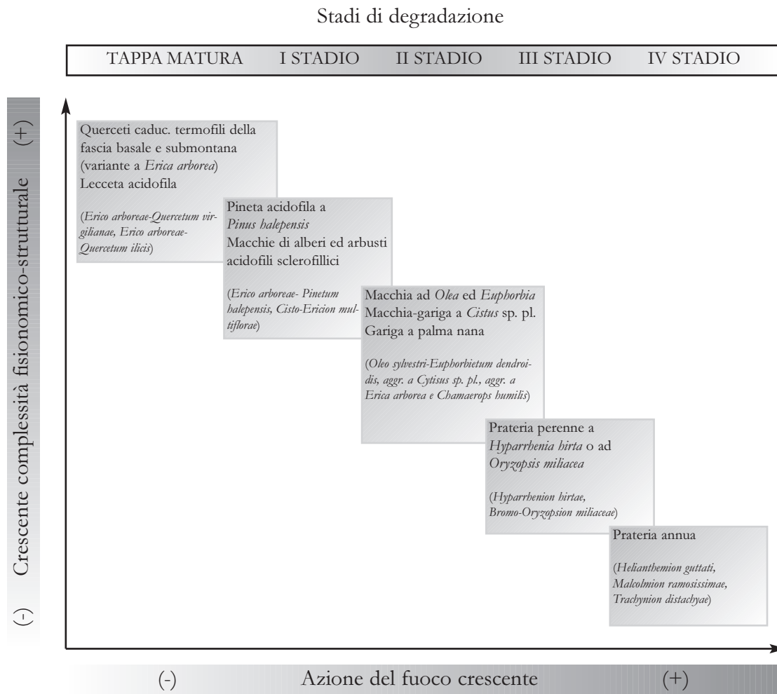
Fig. 8.53 - Schema della dinamica della vegetazione acidofila del piano termomediterraneo delle Eolie (dati da: BRULLO e FURNARI, 1994, aggiornato). La denominazione delle tipologie coinvolte nei diversi stadi della successione segue LA MANTIA et al. (2000, 2001); tra parentesi vengono riportate le corrispondenti unità fitosociologiche. Per la loro ridotta estensione, i lembi di pineta acidofila delle Eolie non sono considerati in LA MANTIA et al. (2000, 2001). Tra parentesi vengono riportate le corrispondenti unità fitosociologiche.
