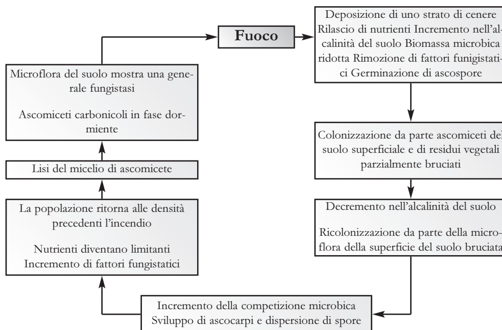
Fig. 2.7 - Relazioni tra fattori biotici ed abiotici associati con il sistema suolo nelle fasi pre- e post-incendio e loro effetto sulla struttura e organizzazione delle comunità di asco.
