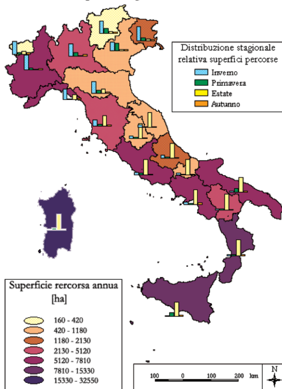
Fig. 4.12 - Stagionalità delle superfici percorse dal fuoco nelle Regioni italiane (anni 1990-2000). Gli istogrammi riportano le frequenze relative nelle stagioni rispetto alla frequenza annua di ogni Regione.
