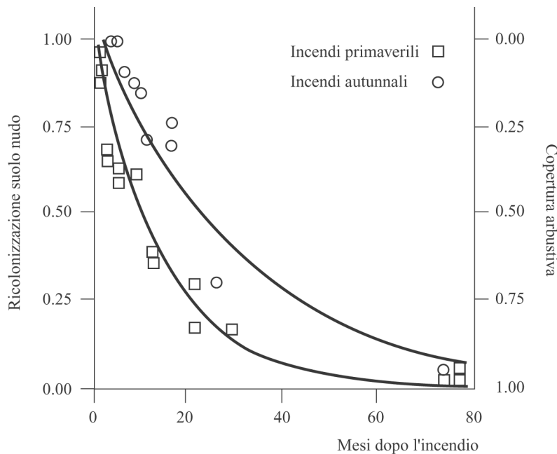
Fig. 8.3 - Influenza della stagione di ricorrenza dell'incendio sull'intensità e velocità di recupero della copertura degli arbusti in una successione post-incendio (da CASAL, 1987).
