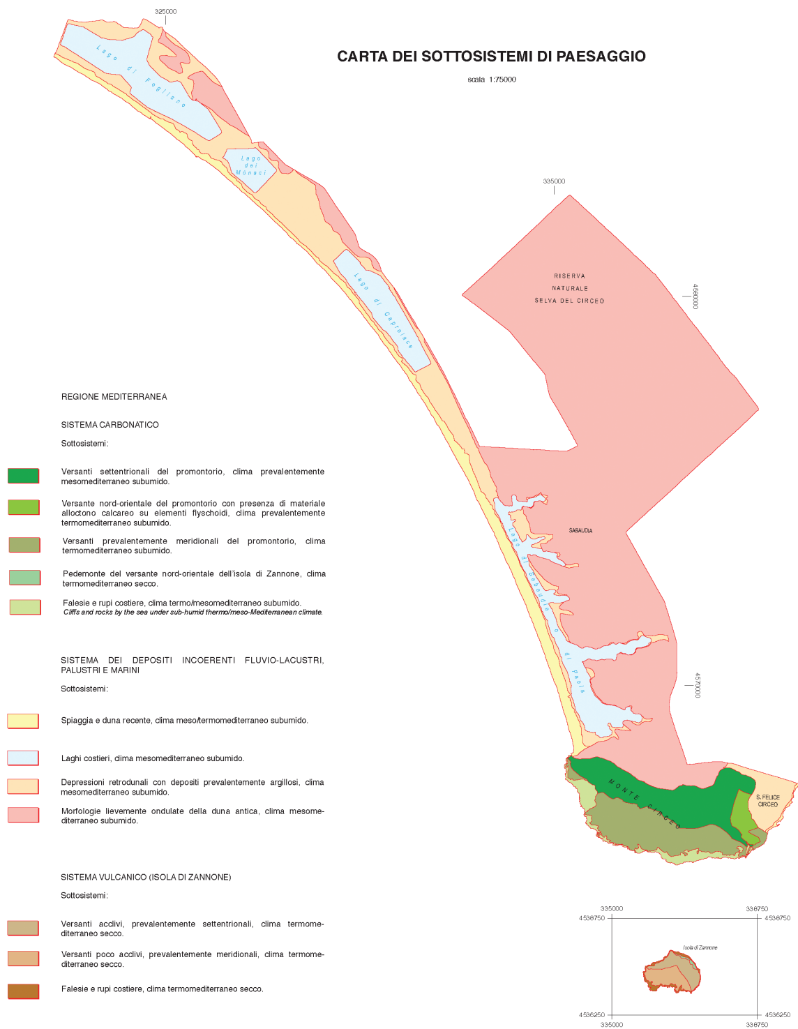
Fig. 8.31 - Classificazione gerarchica territoriale del Parco Nazionale del Circeo.
