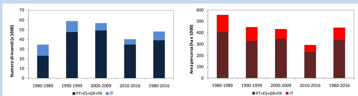
Fig. 15 - Media del numero di incendi (a sinistra) e area percorsa (a destra) in Italia e nel resto del Sud Europa per diversi periodi temporali
